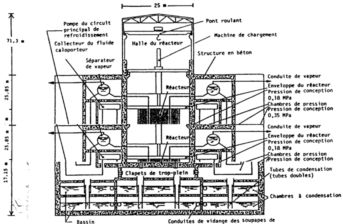
Coupe du bâtiment du réacteur (AIEA).
