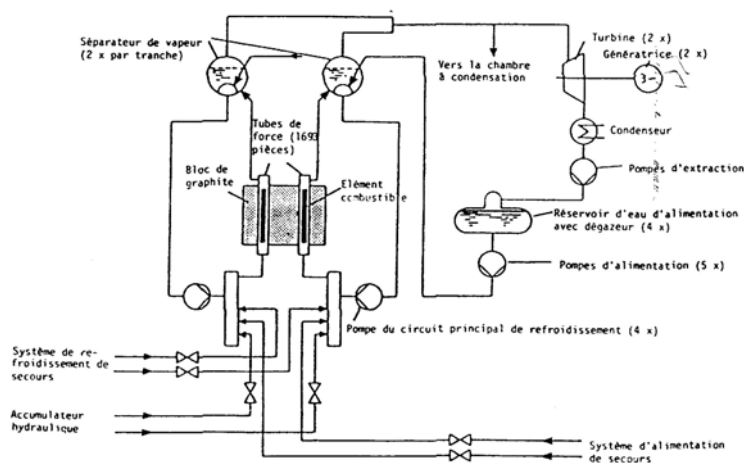
Schéma de principe de la centrale de Tchernobyl.
