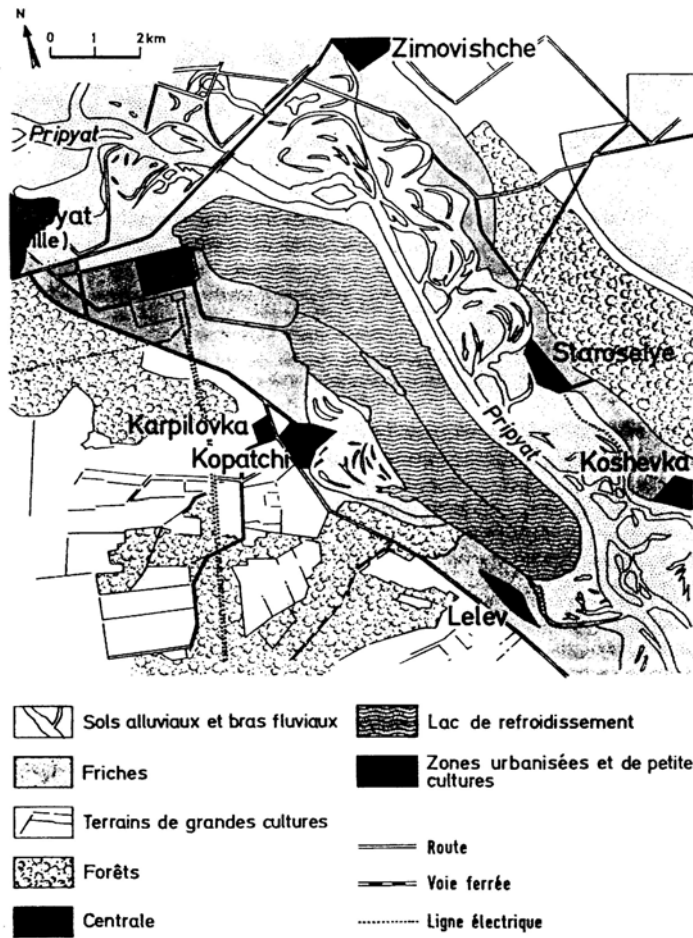
Schéma des environs de la centrale de Tchernobyl (Commissariat à l'énergie atomique).
