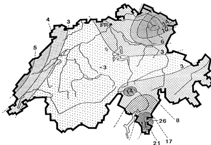
Retombées moyennes de césium 137 en Suisse (valeurs pour le césium 134 \approx valeurs de césium 137 \times 0.6, valeurs pour le iode 131 \approx valeurs de césium 137 \times 7)
